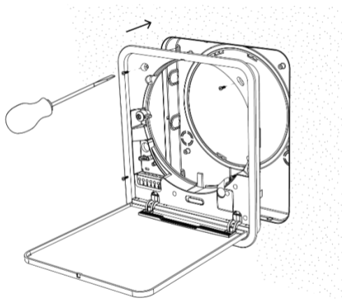
Unterputz Variante
